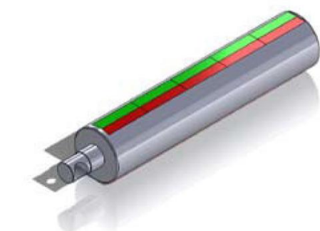
Hagyományos emelőmágnesek Kimart vagy hegesztett kapcsolótengely beszerelt mágnesekkel, 180° elméleti kapcsolási út, legyengített vagy hegesztett tengely, 3 légrés
