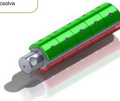
FX emelőmágnesek Tömör kapcsolótengely felcsavarozott mágnesekkel, 90° elméleti kapcsolási út, extrém robusztus, csak egy légrés
